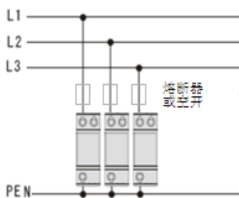
TN-C 三相四线系统 ( KDY-I-50/385/3P )
