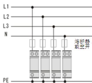
TN-S 三相五线系统 ( KDY-I-50/385/4P )
