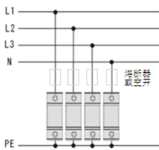
TN-S 三相五线系统 ( KDY-20/320/4P )
