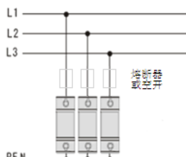
TN-C 三相四线系统 ( KDY-20/320/3P )
