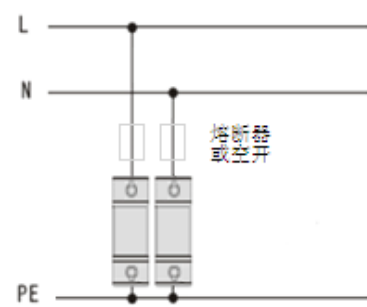
单相三线/二线系统 ( KDY-20/320/2P )
