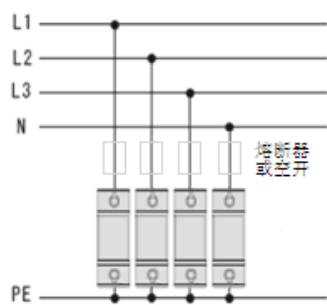
TN-S 三相五线系统 ( KDY-40/440/4P )
