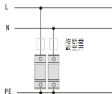
单相三线/二线系统 ( KDY-40/440/2P )
