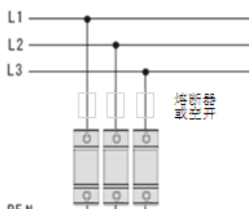
TN-C 三相四线系统 ( KDY-40/440/3P )
