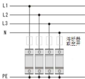
TN-S 三相五线系统 ( KDY-80/385/4P )
