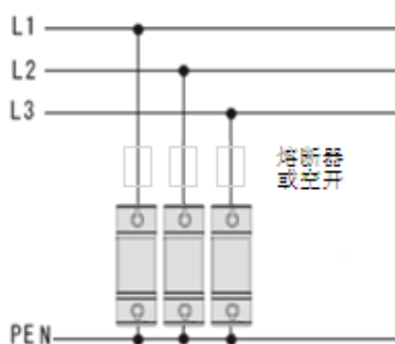
TN-C 三相四线系统 ( KDY-80/385/3P )
