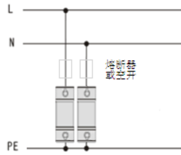
单相三线/二线系统 ( KDY-80/385/2P )
